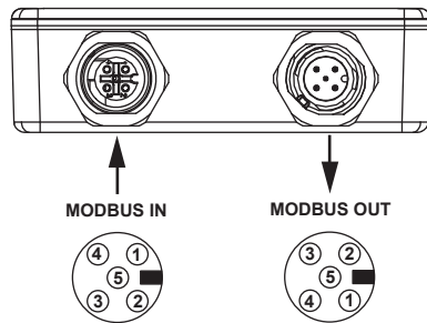
Abb. 5: Anschlussbelegung
